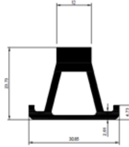
Alüminyum Özel Somun
