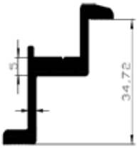
35'lik End Klemp 693 791 gr/m
