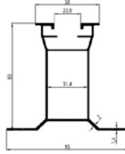
8 cm Aşık Profili 1818 1215 gr/m
