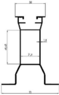
10 cm Aşık Profili 1795 1446 gr/m
