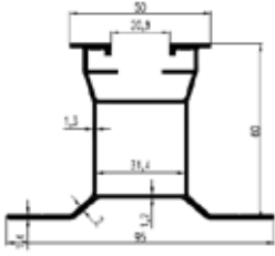
6 cm Aşık Profili 1796 1063 gr/m
