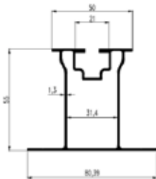
Kulaklı 5,5 cm Aşık 1788 998 gr/m
