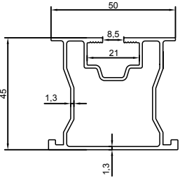
Üst Ray YB-M02 872 gr/m
