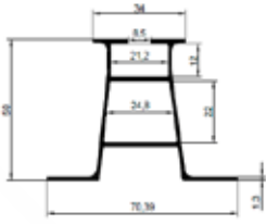
5 cm Kulaksız Aşık Profili 50-3 737 gr/m
