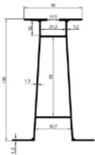
10 cm Aşık Profili 100-1 1143 gr/m
